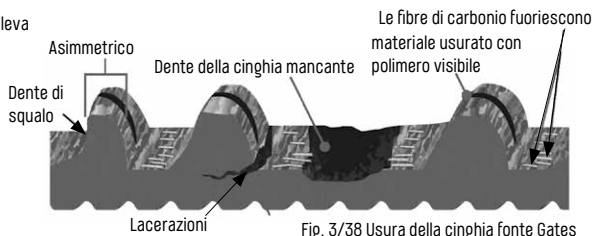
Fig. 3/38 Usura della cinghia fonte Gates
