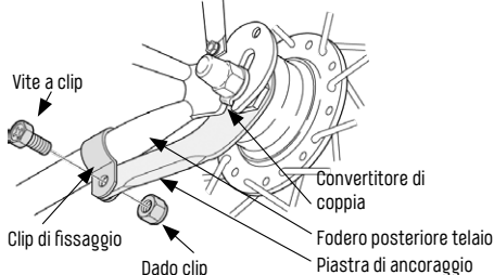
Fig. 3/31 Piastra di ancoraggio Fonte Shimano
