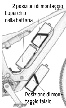
Fig. 1/ Esempi di posizioni di montaggio EPAC
