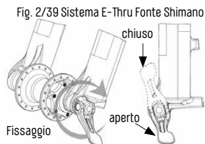
Fig. 2/39 Sistema E-Thru Fonte Shimano
