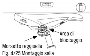
Fig. 4/25 Montaggio sella
