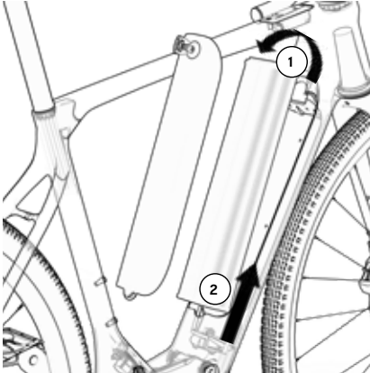
Afb. 3/ Slotzijde boven
