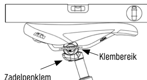
Afb. 4/25 Zadelmontage
