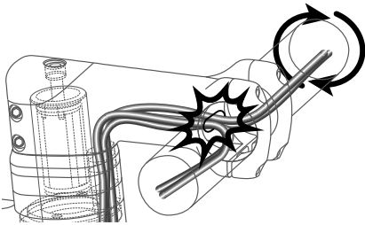
Afb. 1/26 In het frame lopende remleidingen en versnellingskabels
