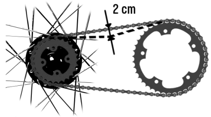
Afb. 4/31 Kettingspanning
