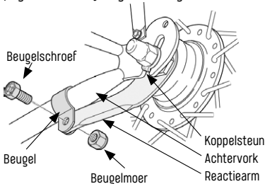
Afb. 3/31 Reactiearm bron Shimano
